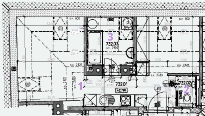
PŮDORYS B.J. 732 1:75
